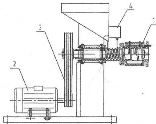
Рисунок 1 – Схема шнекового пресу 1 – вал шнековий, 2 – електродвигун, 3 – привід, 4 – пароутворювач
