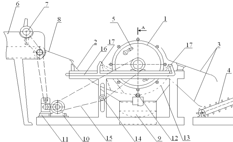
Рис. 8. Машина для виділення насіння дині та огірка:
