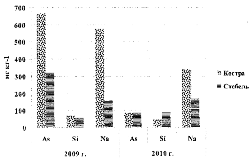
Рис. 3. Содержание мышьяка, силиция и натрия (в сухой массе) в стеблях и костре конопли
