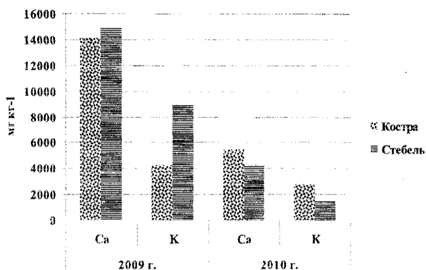
Рис. 2. Содержание кальция и калия (в сухой массе) в стеблях и костре конопли
