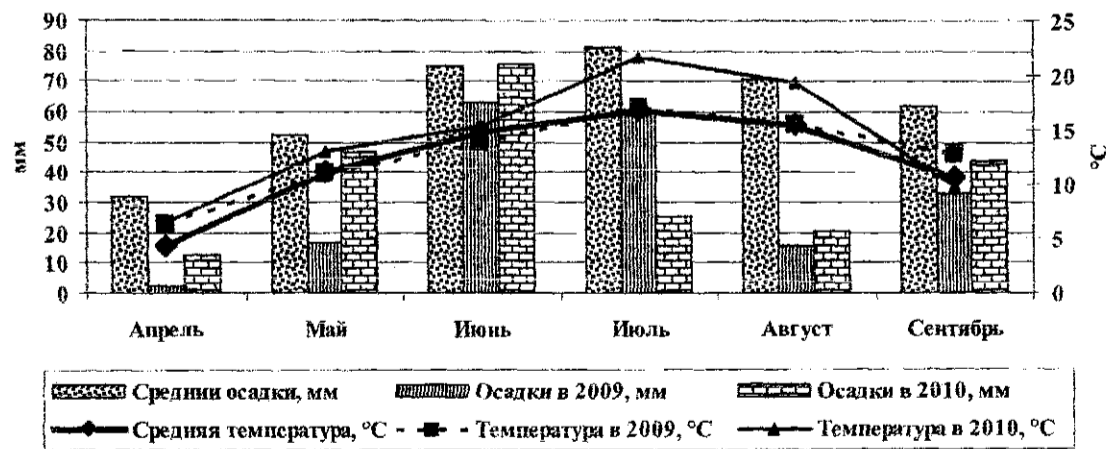
Рис. 1. Характеристика метеорологических условий в годы проведения исследований (Латвия)
