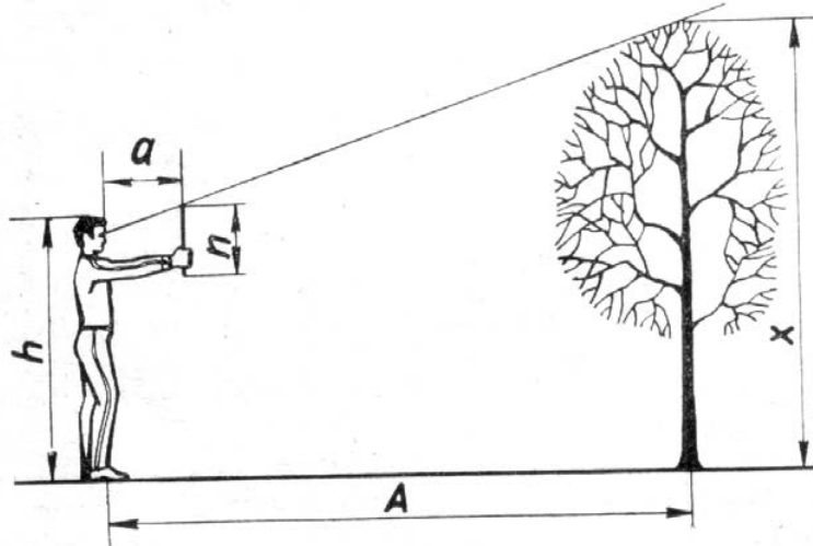
Рис. 10. Окомірне визначення висоти дерев
