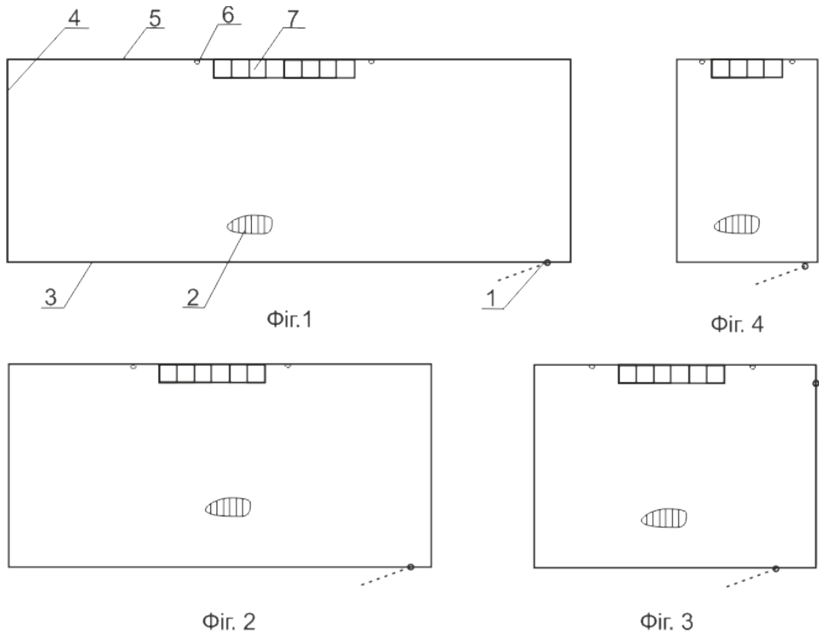
Рис. 3.15. Станки для відгодівлі молодняку свиней: фіг. 1 – станок для 4-х, гнізд, фіг. 2 – станок для 3-х гнізд, фіг. 3 – станок для 2-х гнізд, фіг. 4 – станок для одного гнізда. Експлікація станка: 1 – дверцята, 2 – решітчаста підлога, 3 – задня огорожа, 4 – бокова огорожа, 5 – передня огорожа, 6 – чашкова автонапувалка, 7 – бункерна самогодівниця
