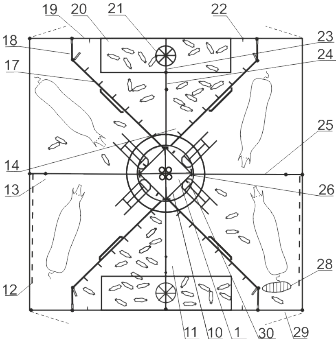
Рис. 3.10. Станок після розфіксації свиноматки
